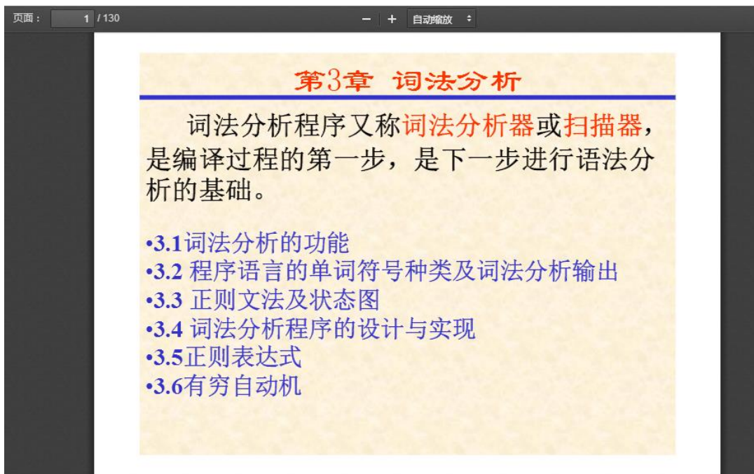
图 5 “查看”资源
