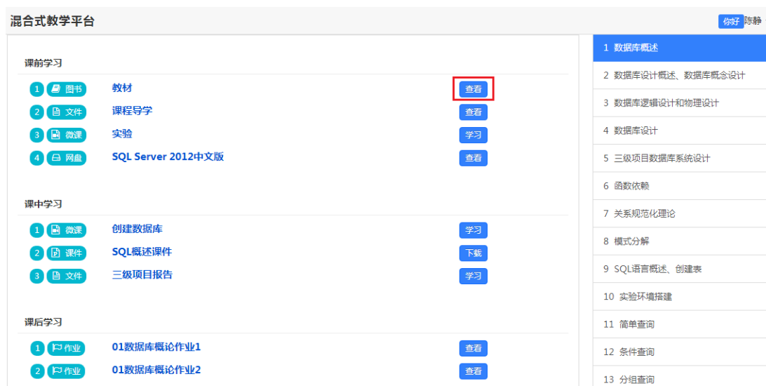
图 4 学习页面
